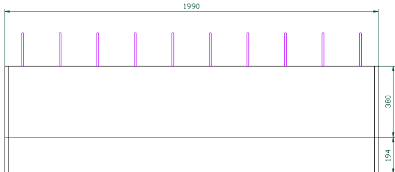
Armado imposta , cercos y varillas corrugadas B500S
